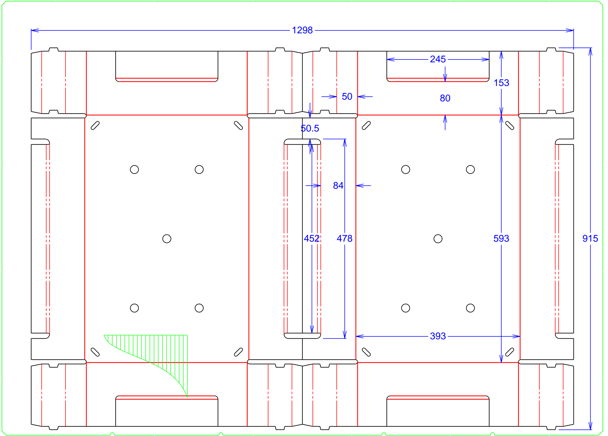
PINZA LATO STAMPA IC6609
