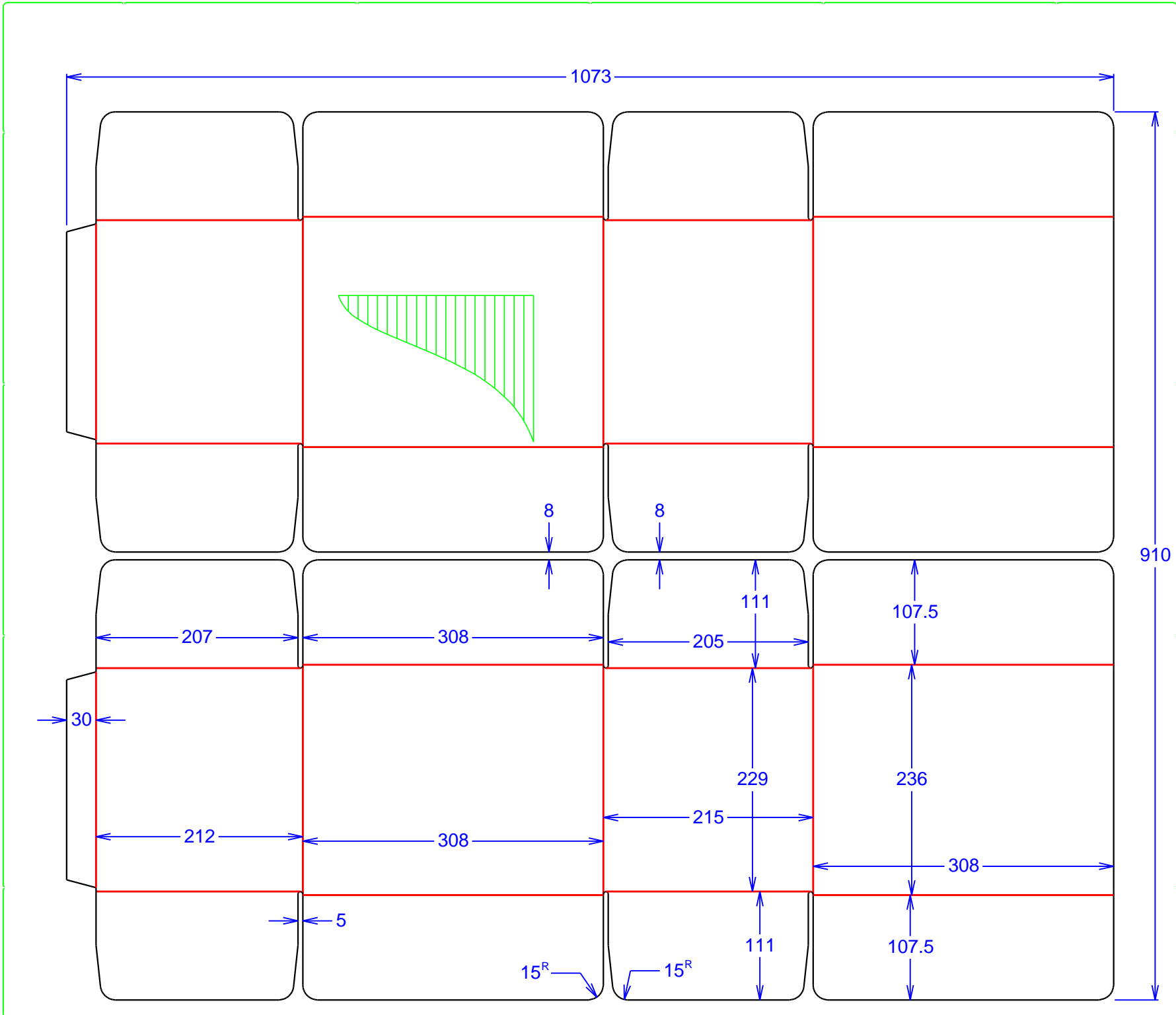
PINZA LATO STAMPA NLB369
